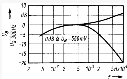
Bild 3. Frequenzgang des Verstärkers mit dem Netzwerk nach Bild 2
