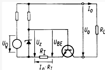
Bild 6. Grundsaltung für Stromstabilisierung
