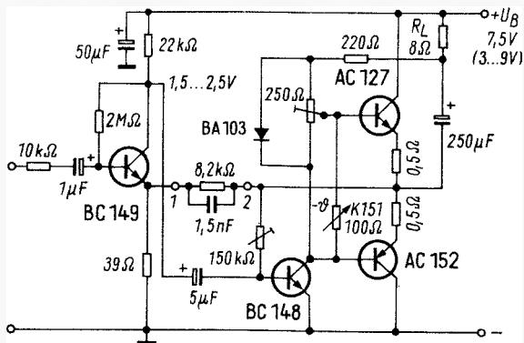
Links: Bild 1. Schaltung des Nf-Verstärkers
