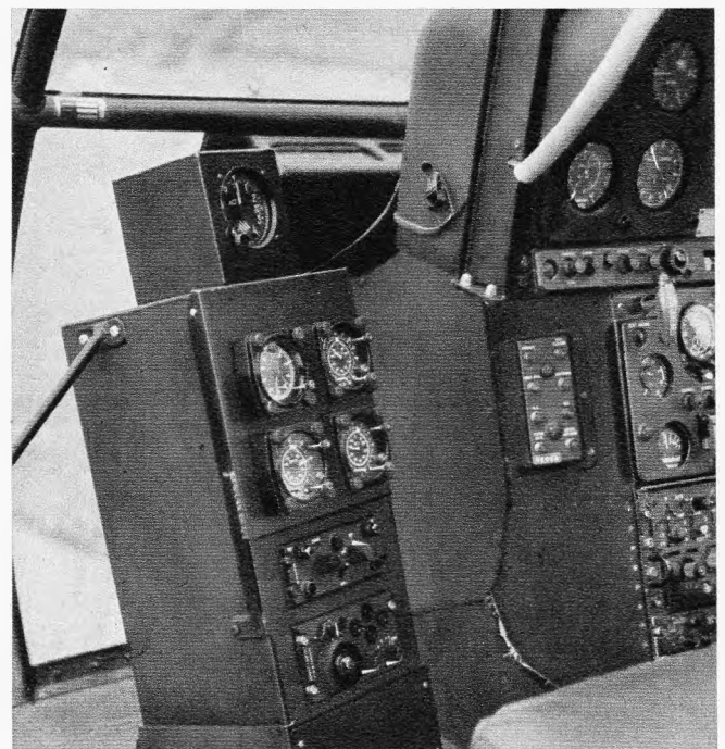
Bild 6. Das Decca-Bedienungsgerät
