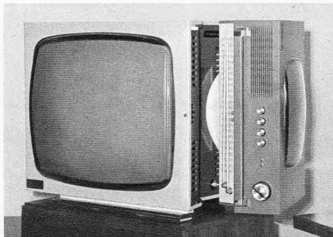
Rechts: Bild 2. Kombinationsfernsehgerät Diamond, zusammengesetzt aus einem 31-cm-Portable und einem 61-cm-Bildschirm. Zum Betrieb des größeren Bildes müssen beide Teile zusammengesteckt werden
