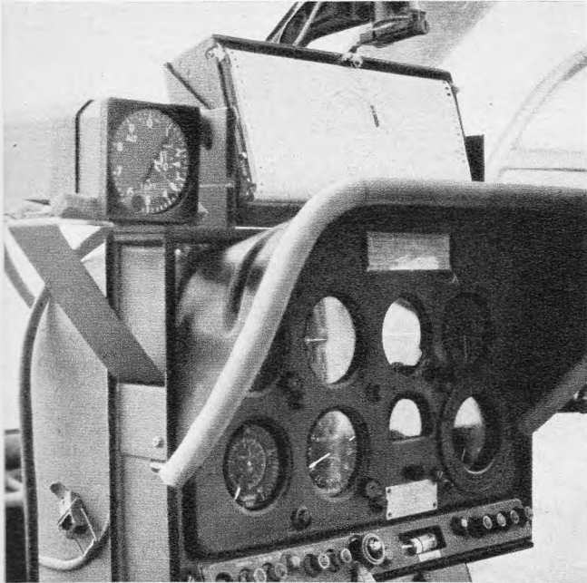
Bild 7. Der Flugwegschreiber. Sein Schreibstift bewegt sich in X-Richtung, die Karte in Y-Richtung
