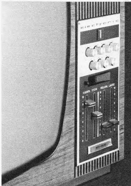
Bild 6. Abstimmteil der Grundig-Farbfernsehgeräte mit sieben Stationstasten und Schiebepotentiometern sowie Leuchtzifferanzeige des gewählten Programms
