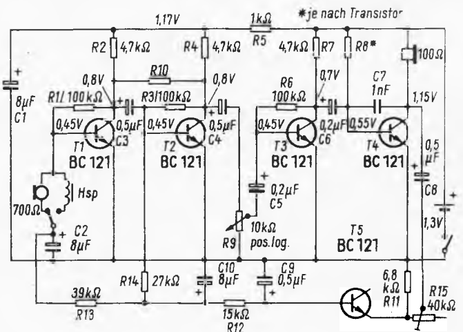
Rechts: Bild 13. Vierstufiger Hörgeräteverstärker mit AVC und Hörschleife. Wert von R 8 je nach Transistor (Siemens)
