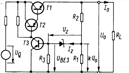
Bild 14. Betrieb der Z-Diode mit fast konstantem Strom. U_z hat einen kleinen Temperaturgang
