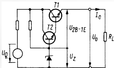
Bild 5. Anwendung der Darlington-Schaltung im Stellglied zur Erhöhung der Regelsteilheit
