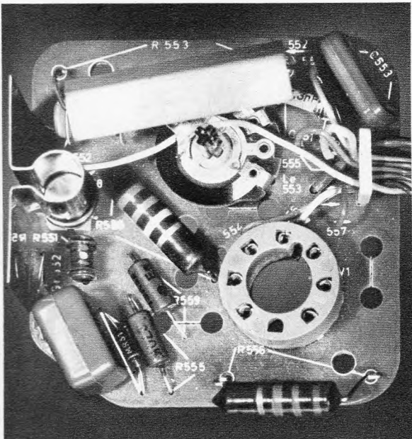
Bild 10. Bildröhrenplatte im Chassis F 209 von AEG-Telefunken mit Video-Endstufe (Transistoren im Kühlblech)
