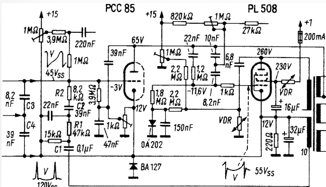
Ein Fehlen des positiven Rückschlagimpulses am Steuergitter der Röhre PCC 85 war die Ursache für eine verringerte Vertikaloszillationsfrequenz
