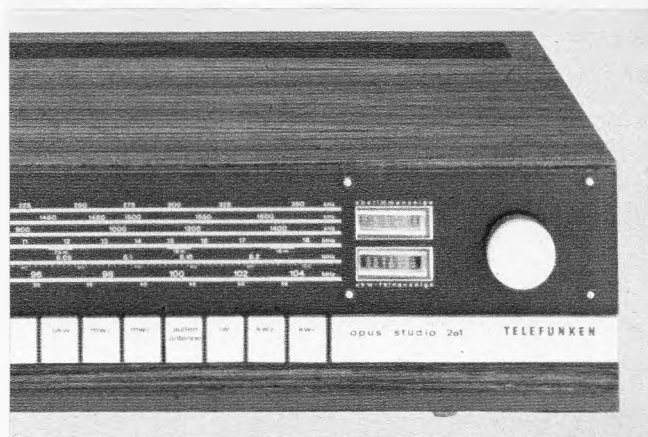
Bild 5. Der Telefunken-Opus hat zwei Instrumente für die Abstimmung. Das untere arbeitet auch für die erwähnte Übernahmestelle. Ein drittes, nicht sichtbares, in MHz geeichtes Instrument gehört zu den Stationstasten
