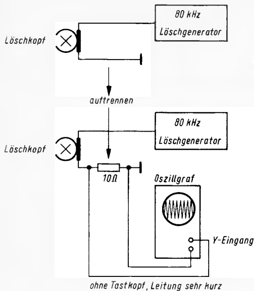
Bild 22. Indirekte Strommessung mit einem Oszillografen
