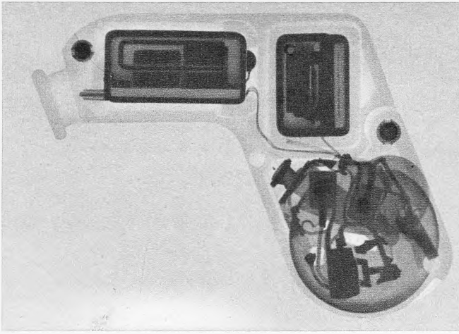
Bild 25. Röntgenaufnahme eines IdO-Gerätes (Siemens)
