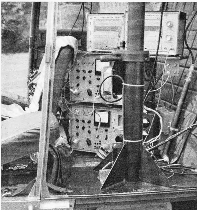
Bild 5. Geräteausrüstung des Hubschraubers, Teleskopmast mit Meßantenne
