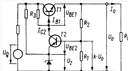
Bild 7. Erweiterte Schaltung für Spannungsstabilisierung. Der Transistor T2 dient zur Verstärkung der Stellgröße, außerdem ist in das Vergleichsglied ein Spannungsteiler eingeschaltet
