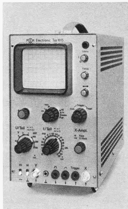
Gleichspannungsozillograf, Typ 1015, von PEK-Electronic, mit einer Bandbreite von 0...12 MHz. Das Gerät ist triggerbar
