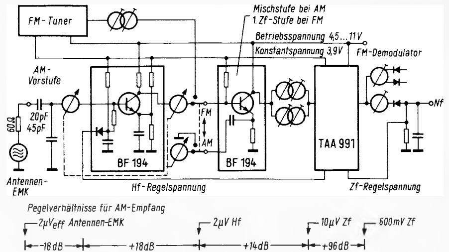
Bild 2. Blockschaltung eines AM/FM-Empfängers mit der integrierten Schaltung TAA 991 von Siemens
