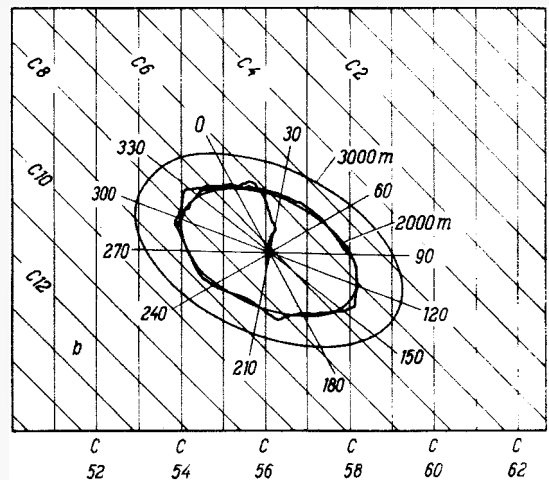
Bild 8. Flugwegkarten verschiedener Senderstandorte; oben für den Sender Torfhaus (125 km Entfernung zur deutschen Decca-Kette); unten für den Sender Pforzheim (325 km Entfernung zur deutschen Decca-Kette)
