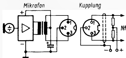
Links: Bild 4. Prinzip der Phantomspeisung eines Kondensatormikrofon
